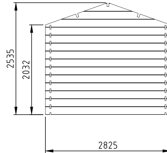
Achterwand 28 dik DOUGLAS WDB03-283 1x
