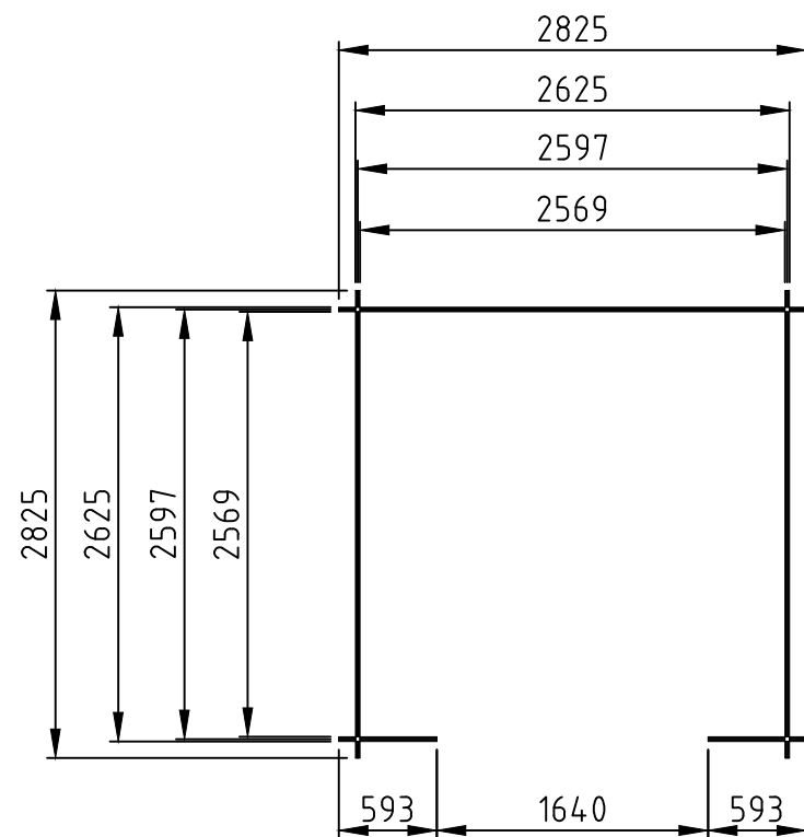
Fundatie gegevens
