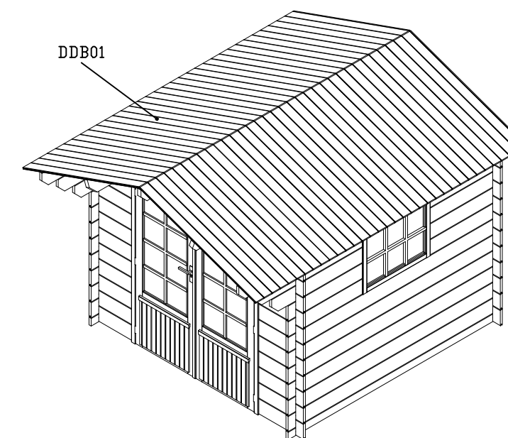
Dakplanken plaatsen.
