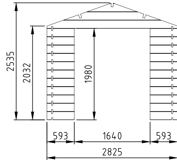
Voorwand 28 dik DOUGLAS WDB01-283 1x
