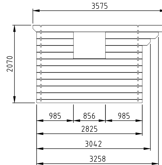
Zijwand met raam 28 dik DOUGLAS WDB04-283 1x
