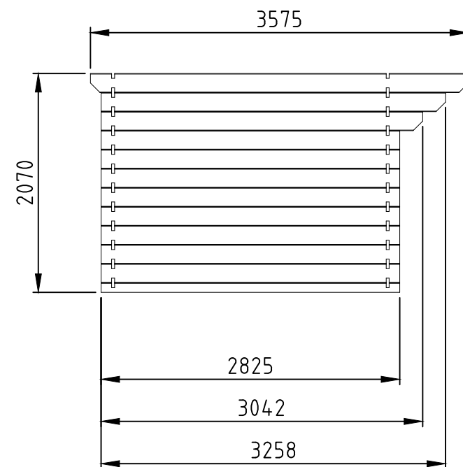
Zijwand dicht 28 dik DOUGLAS WDB05-283 1x
