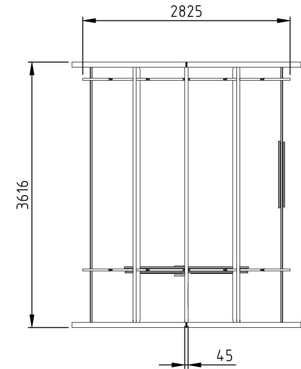
Overzicht gordingen
