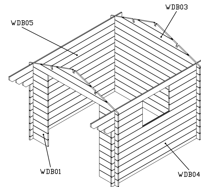
Gevelpunten plaatsen.
