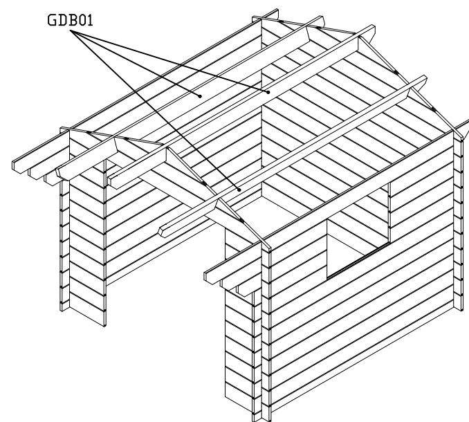
Gordingen plaatsen.
