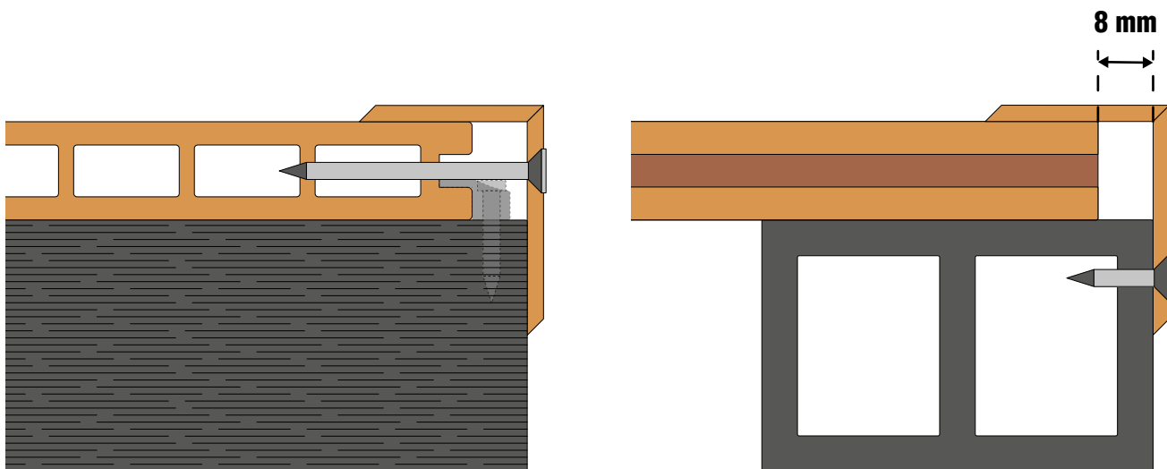
Abb 4: Abschlussarbeiten (Kantenabschluss)
